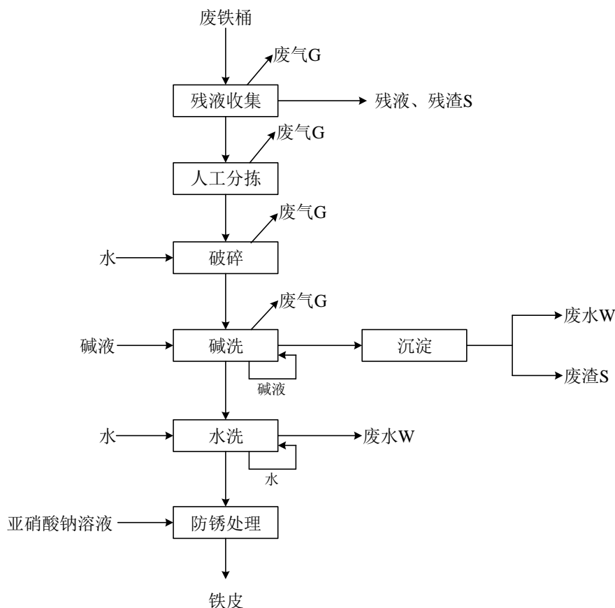
图3.2.7.7-1 废铁桶综合利用工艺流程图及产排污节点
