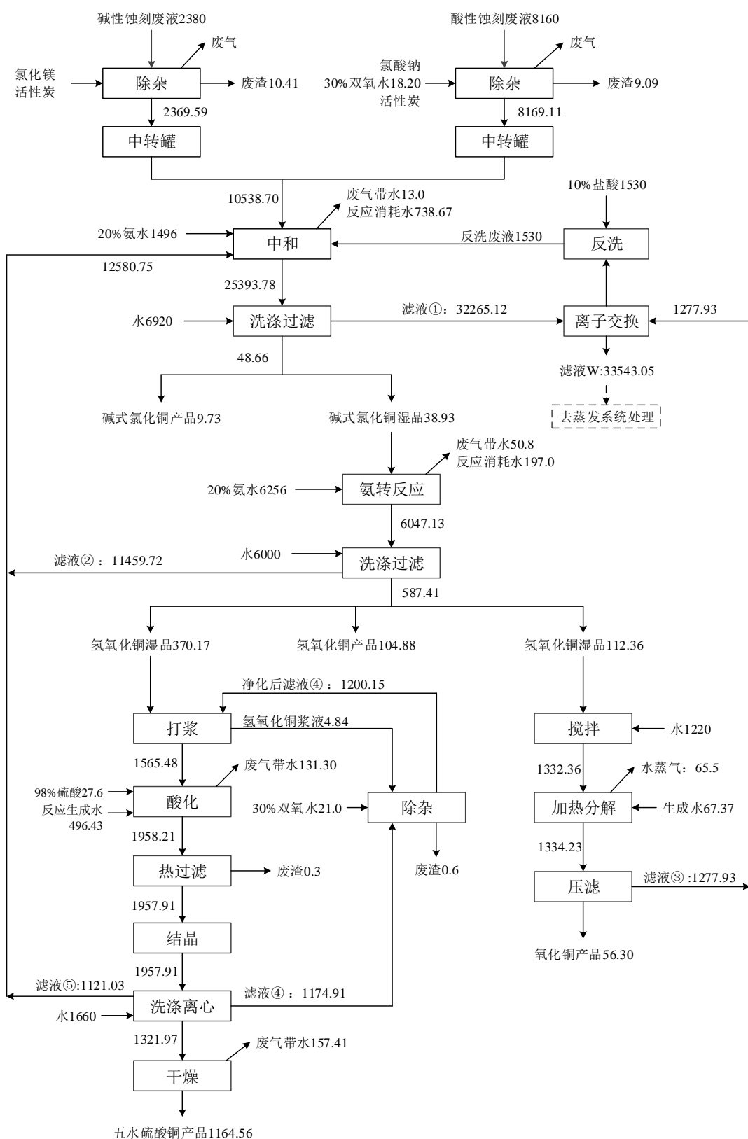
图3.2.7.5-3 技改后含铜蚀刻废液综合利用的水平衡 单位: m³/a
