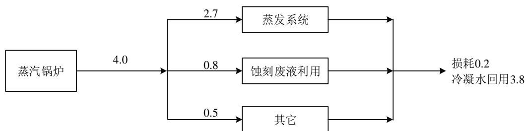
图3.2.4.5-1 技改后全厂蒸汽平衡 单位：t/h
