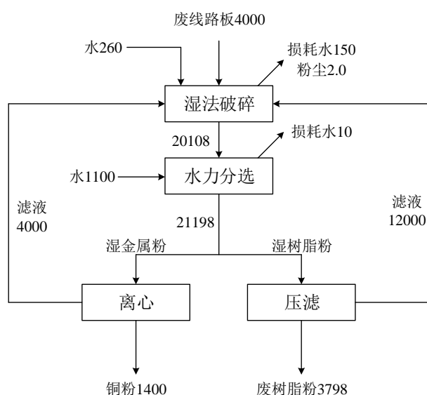
图3.2.7.6-2 技改后废线路板综合利用物料平衡（单位：t/a）
