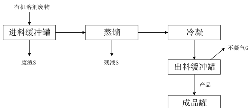
图3.1.6-8 技改前废有机溶剂利用工艺流程及产污节点
