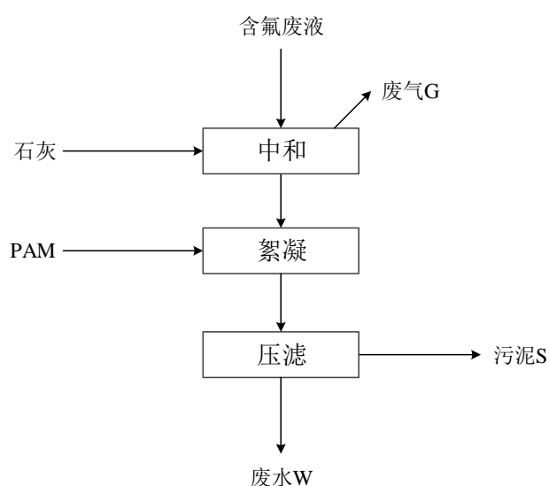
图3.2.7.8-7 含氟废液处理线工艺流程及产污节点
