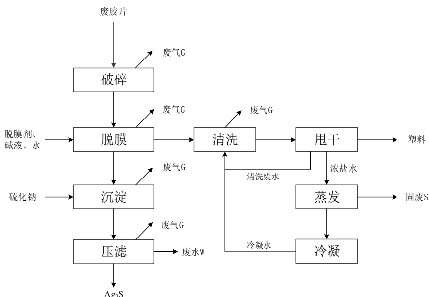
图3.1.6-6 技改前废胶片利用工艺流程及产污节点
