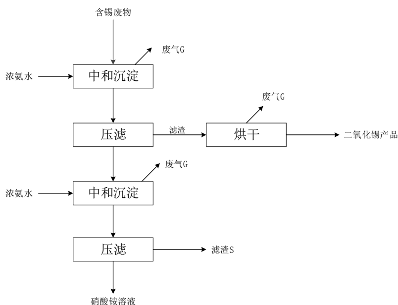
图3.1.6-4 技改前退锡废液利用工艺流程及产污节点
