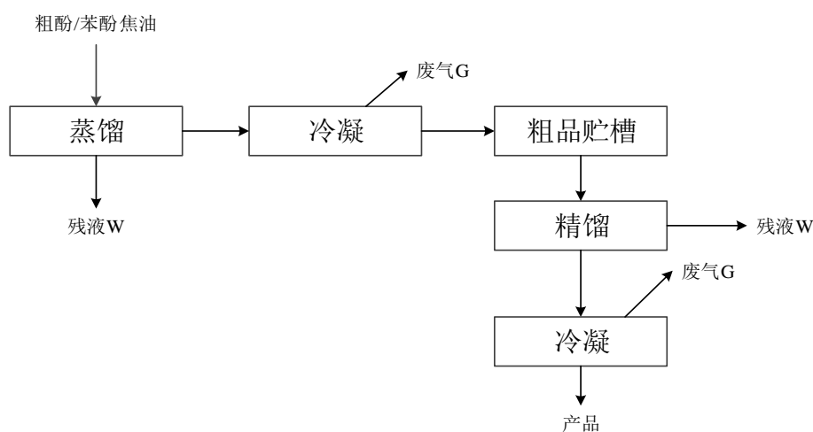
图3.1.6-9 技改前粗酚及苯酚焦油利用工艺流程及产污节点
