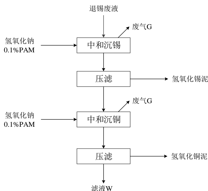
图3.2.7.8-3 退锡废液利用工艺流程及产污节点
