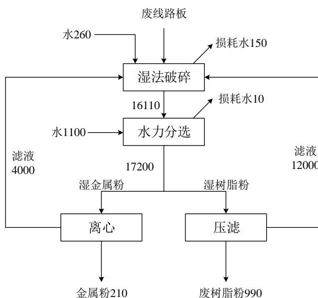
图3.2.7.6-3 技改后废线路板综合利用的水平衡图（单位：t/a）
