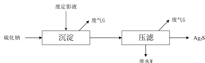
图3.1.6-5 技改前废定影液利用工艺流程及产污节点
