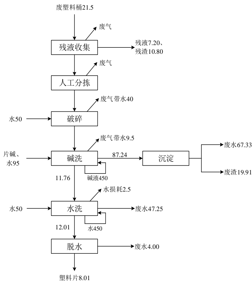
图3.2.7.7-4 废塑料桶综合利用的水平衡 单位：m 3 /a
